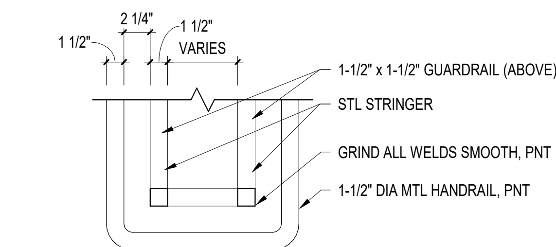
A4 STAIR DETAIL (TYP) SCALE: 1 1/2" = 1'-0" (AE444)
