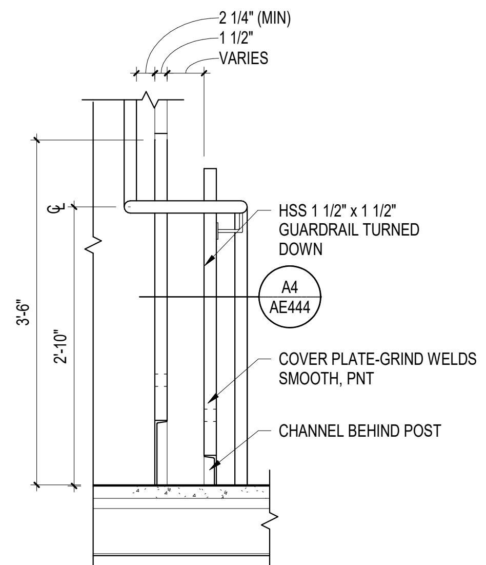
A5 STAIR RAILING ELEVATION (TYP) SCALE: 1" = 1'-0" (AE444)
