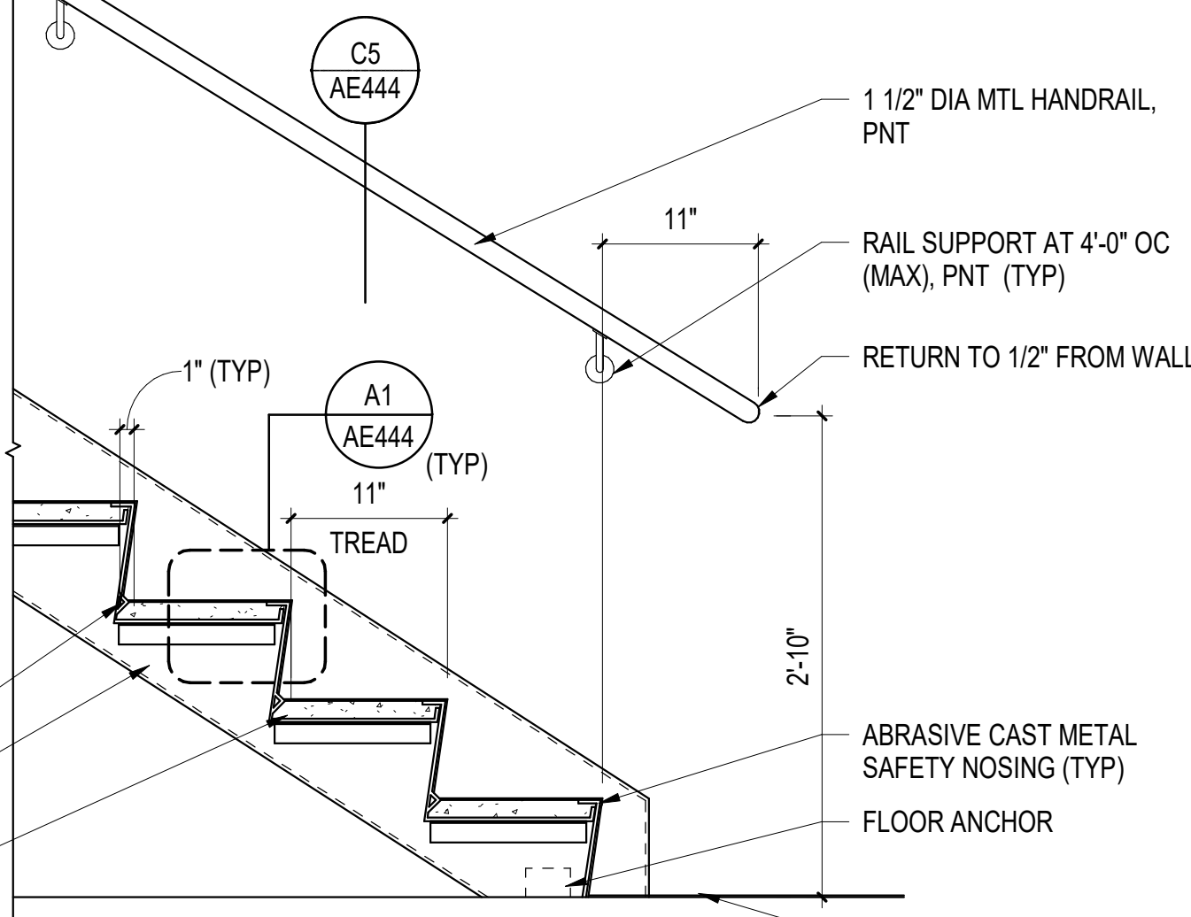
A3 STAIR RUN DETAIL (TYP) SCALE: 1" = 1'-0" (AE442)
