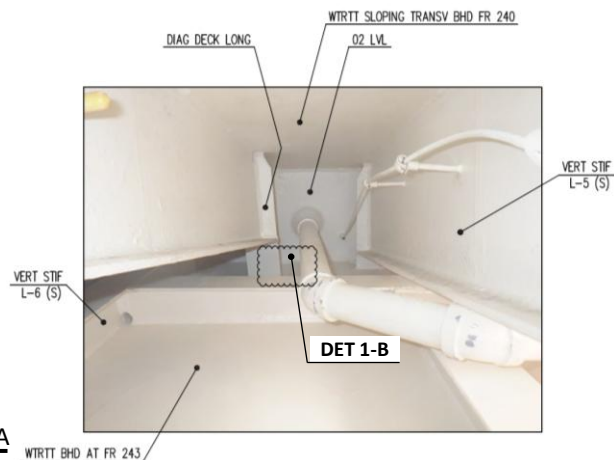
PLAN 1-A 02 LVL DK, FR 241-243 LKG OVHD
