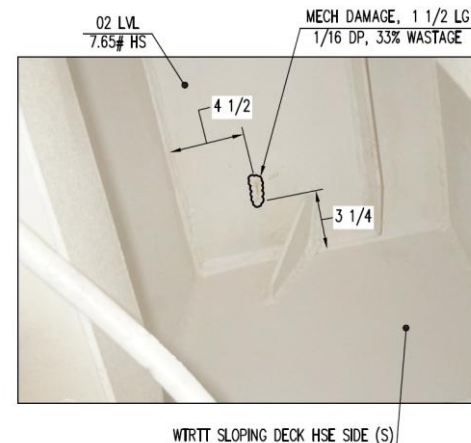
DET 1-D MECH DAMAGE ON 02 LVL DK PLTG
