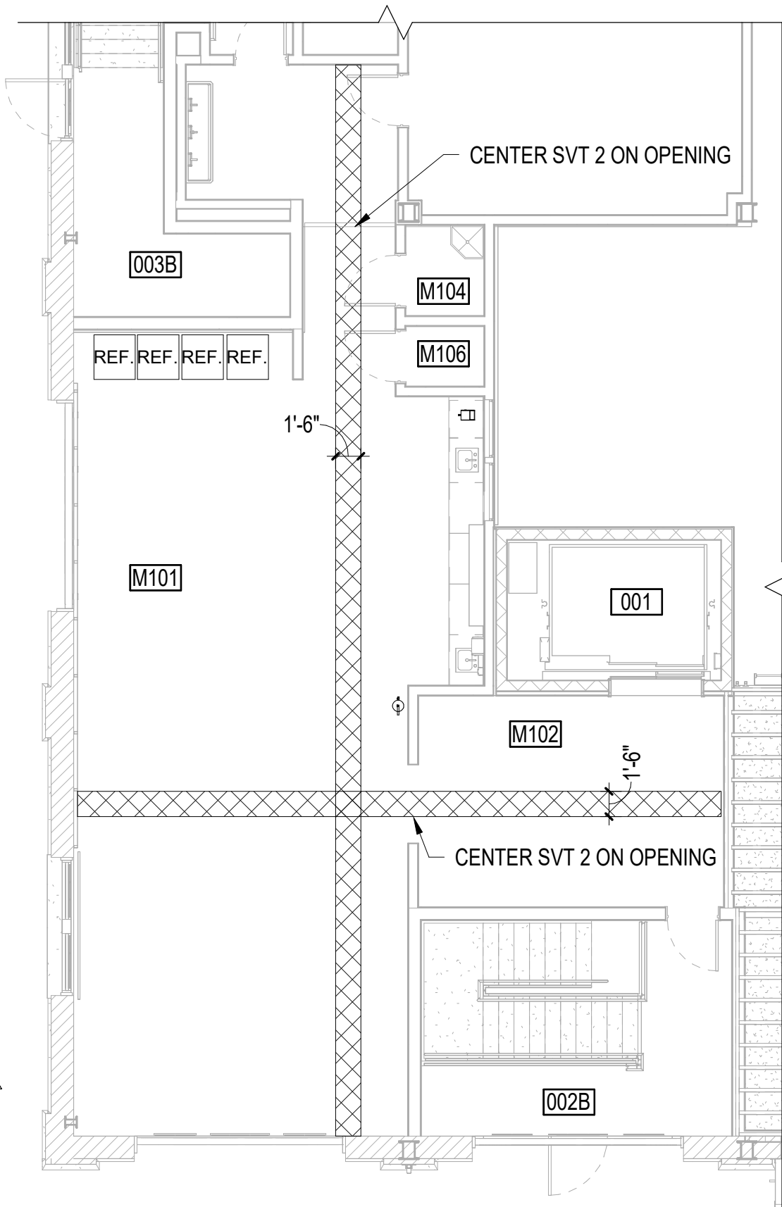
A5 BREAK ROOM M102 FLOOR PATTERN SCALE: 1/8" = 1'-0" (AE104)
