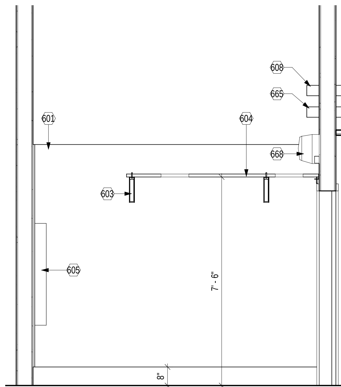
A3 TELECOM 105 - WEST ELEVATION 1/2" = 1'-0" (T-102)
