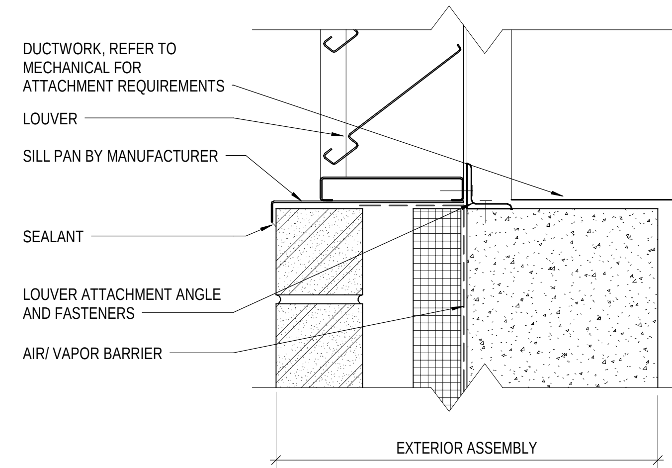
A3 EXT LOUVER SILL DETAIL 3" = 1'-0"
