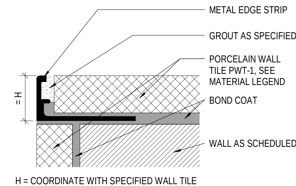
A4 METAL EDGE STRIP DETAIL 12" = 1'-0"
