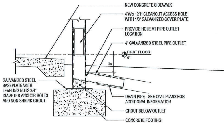
A5 DOWNSPOUT SECTION SCALE: 1" = 1'-0"
