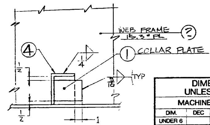
DETAIL 6-A (TYP) 3=1'-0
