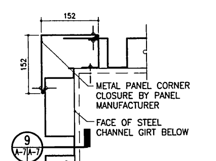
PANEL DETAIL TYP 5
