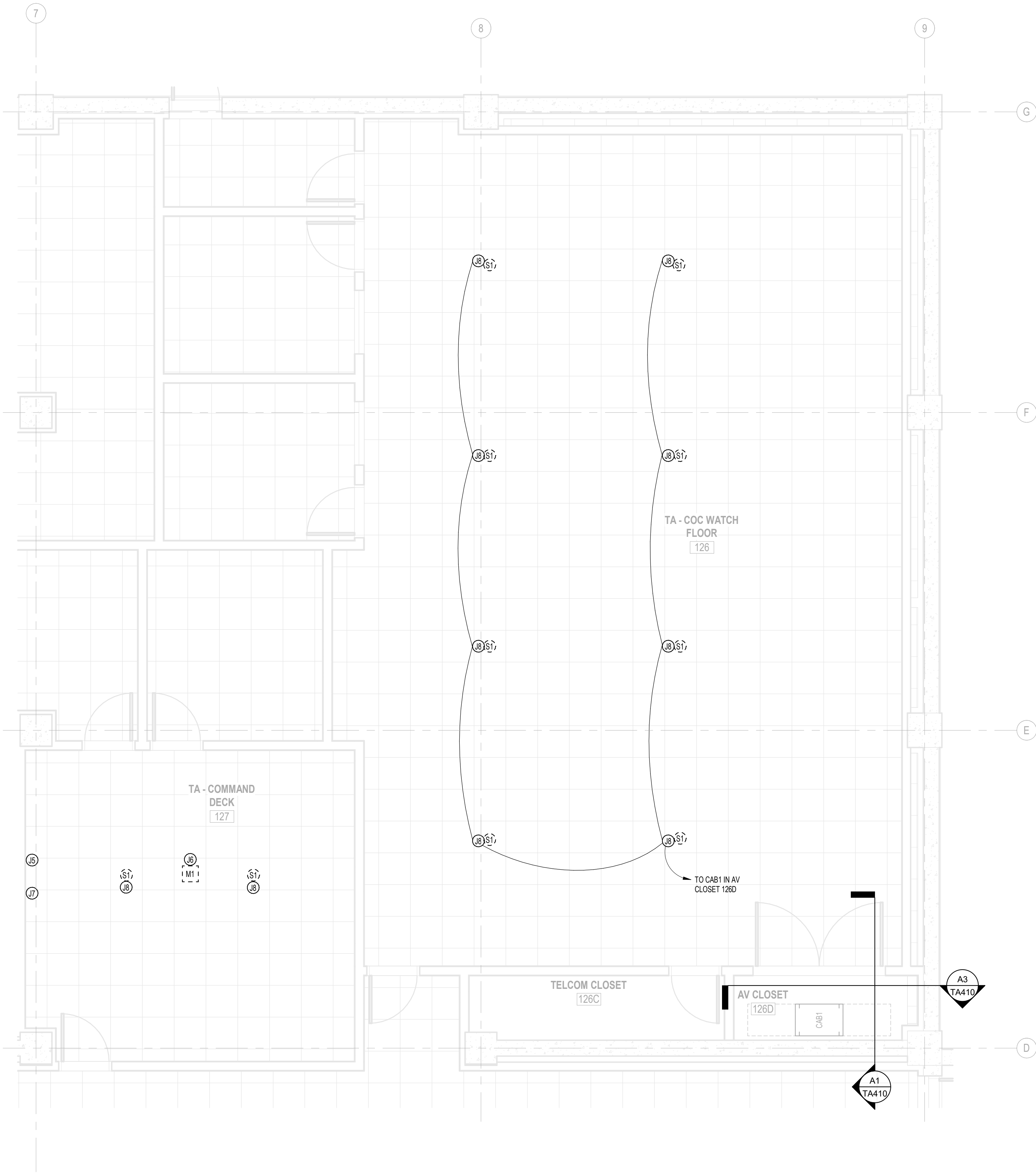
A1 ENLARGED AV SYSTEMS REFLECTED CEILING PLAN - ROOM 126 1/4" = 1'-0"
