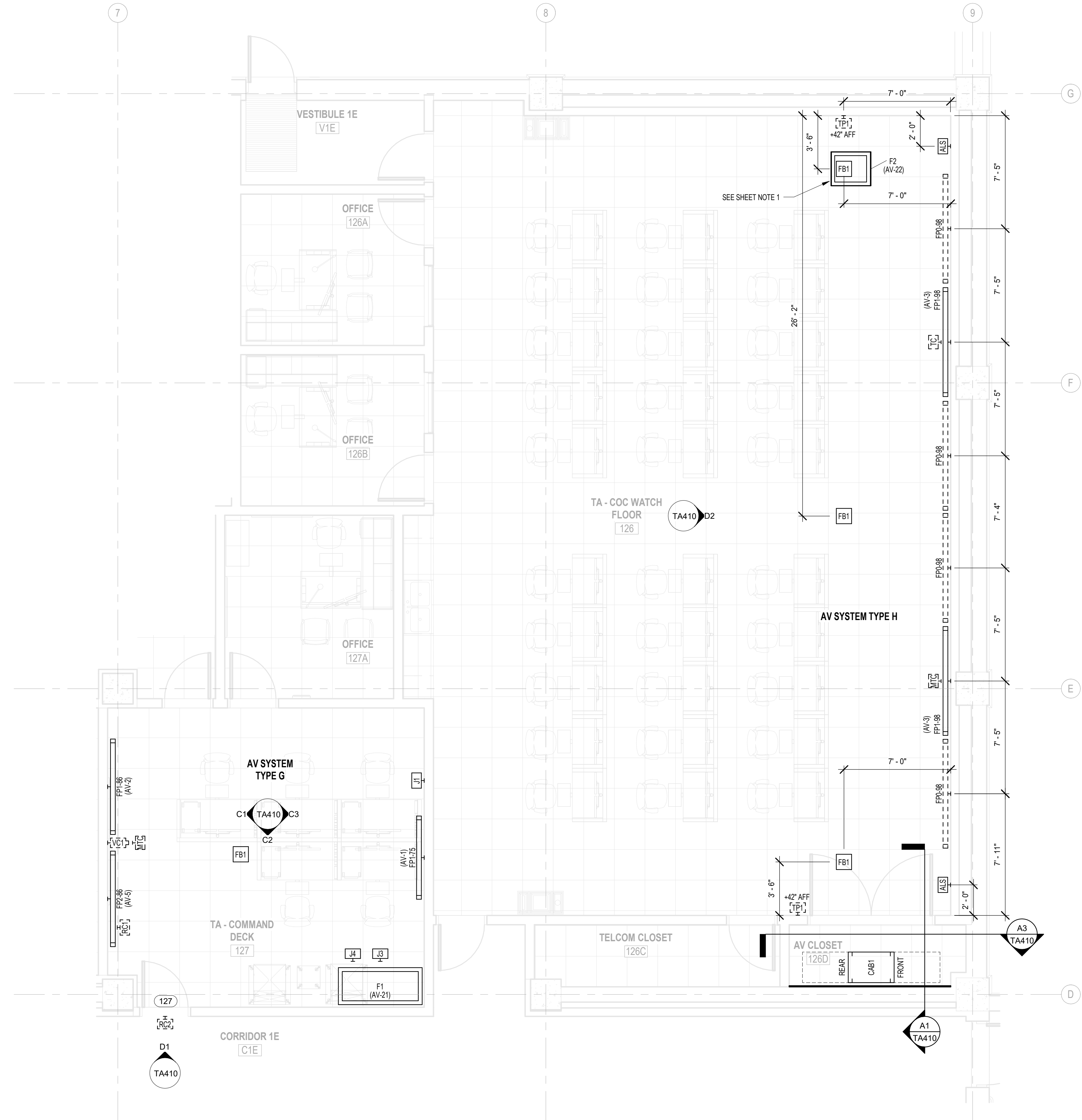
ENLARGED AV FLOOR PLAN TA COC WATCH FLOOR 126 & TA COMMAND DECK 127
