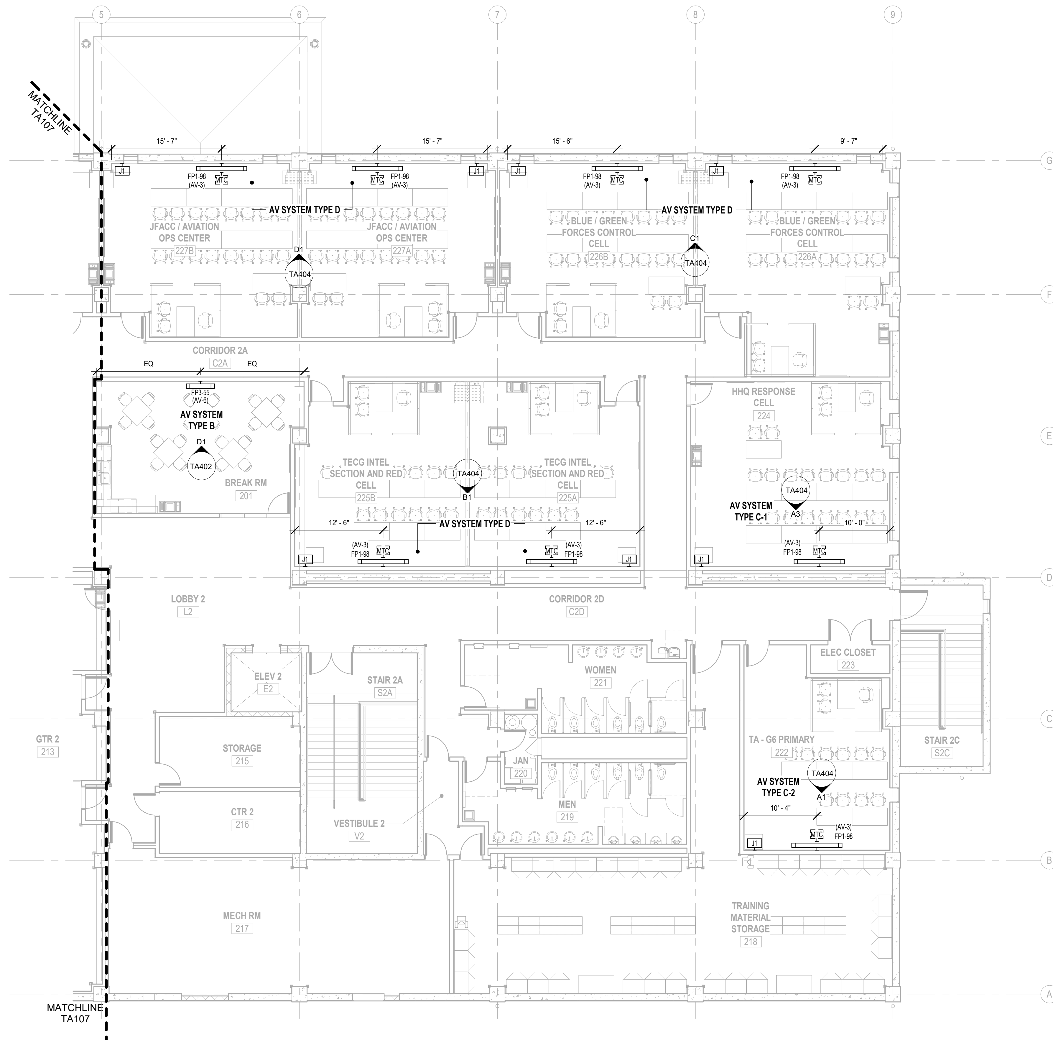
A1 AV SYSTEMS SECOND FLOOR PLAN - B 1/8" = 1'-0"
