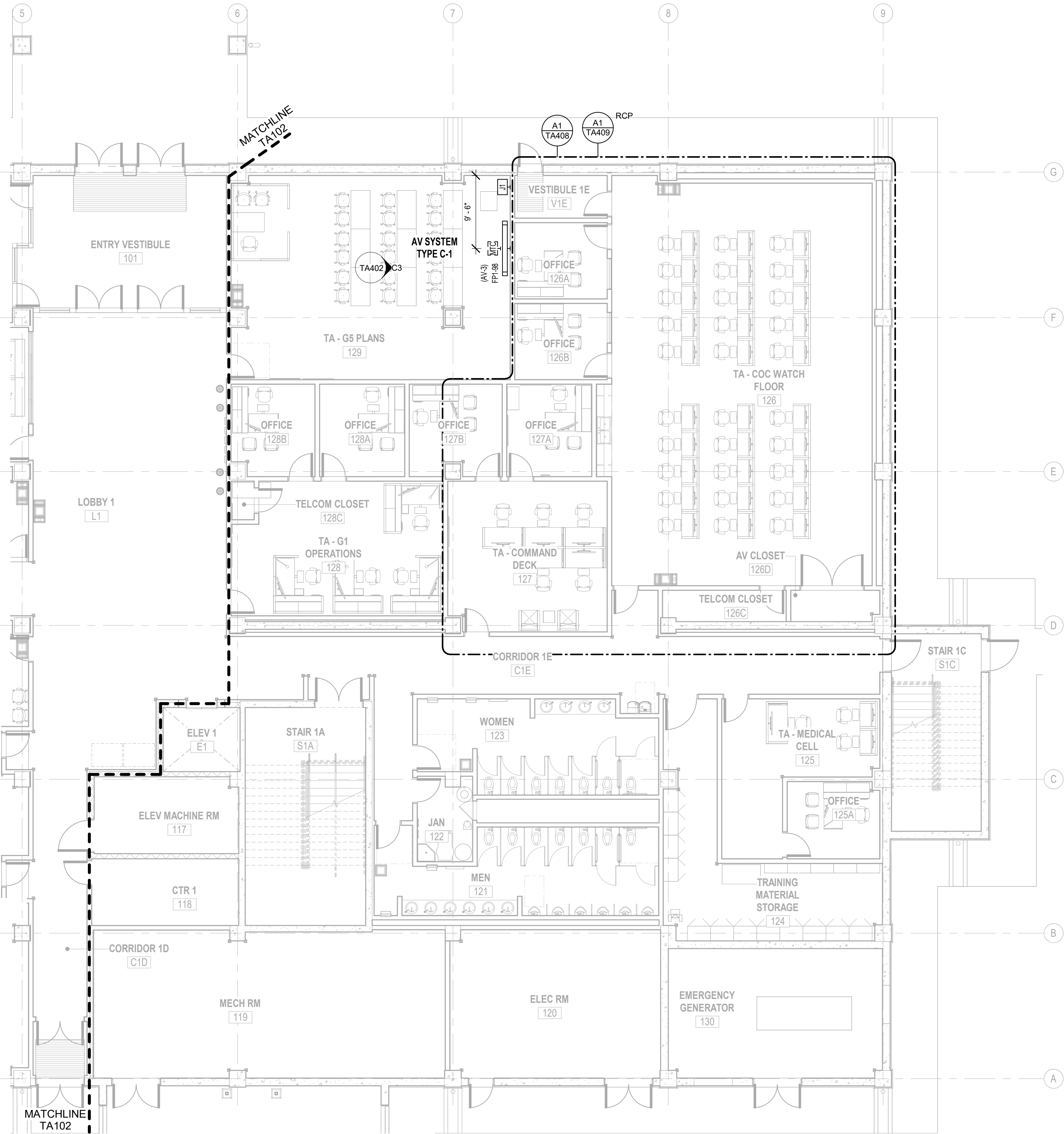
A1 AV SYSTEMS FIRST FLOOR PLAN - B 1/8" = 1'-0"
