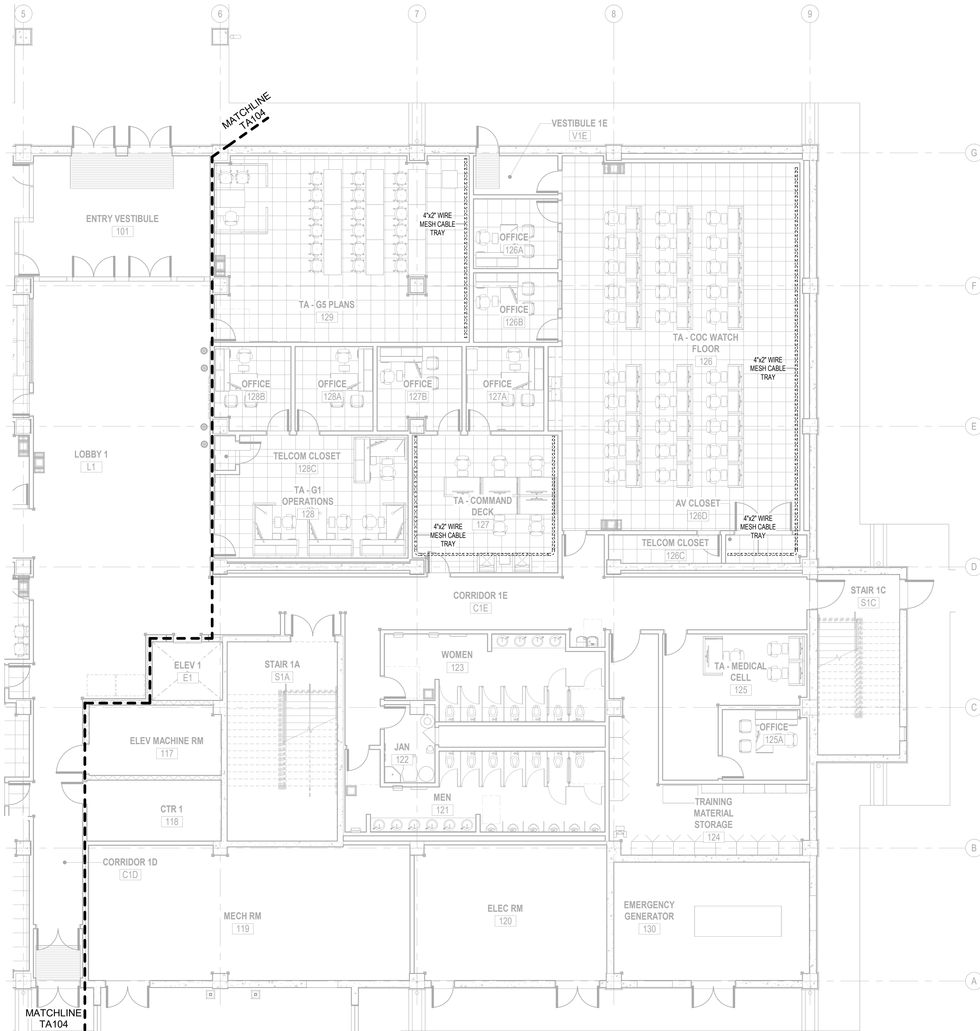
AV UNDER-RAF CABLE TRAY FIRST FLOOR PLAN - B 1/8" = 1'-0"
