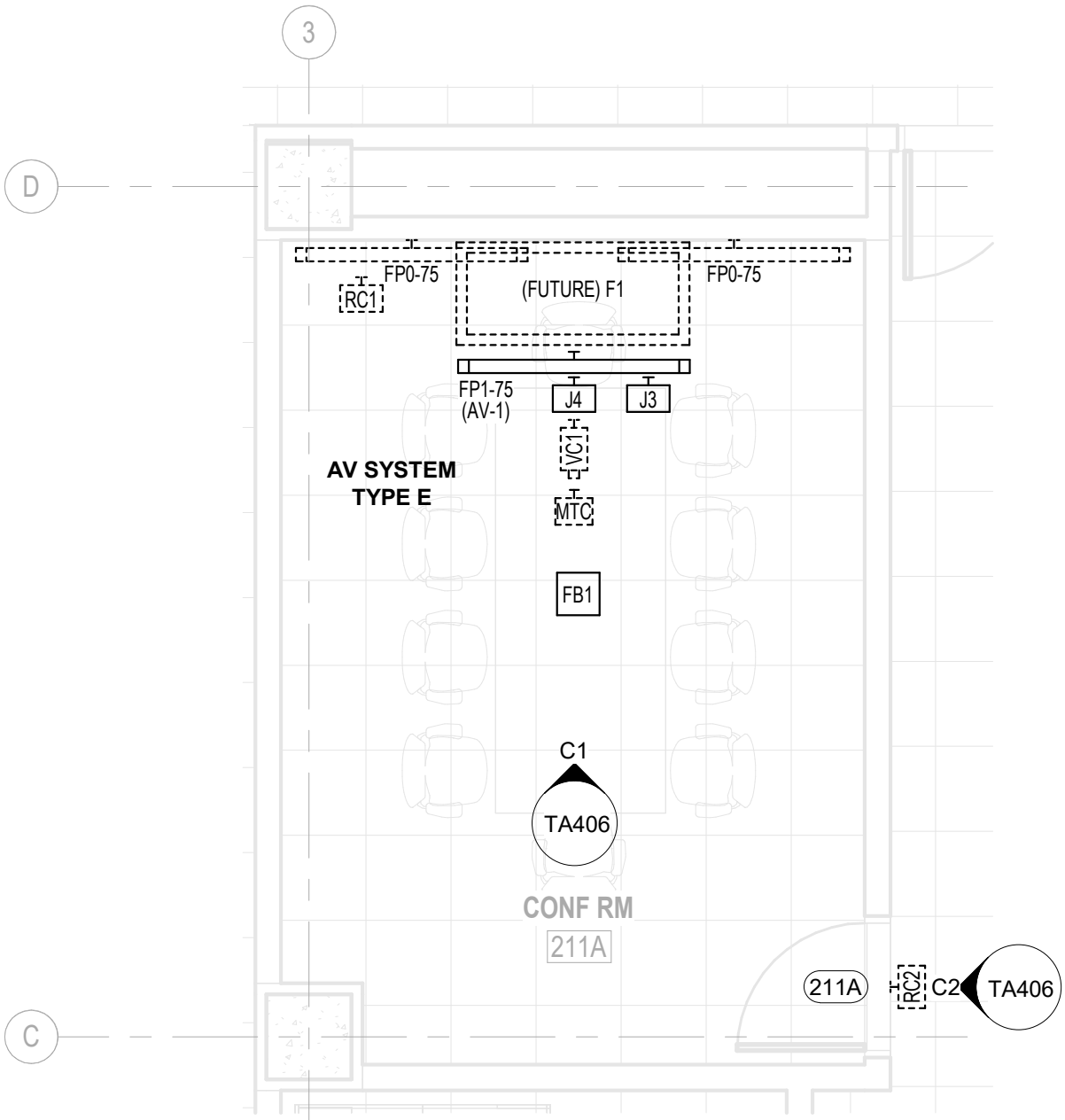
ENLARGED AV FLOOR PLAN CONF RM 211A
