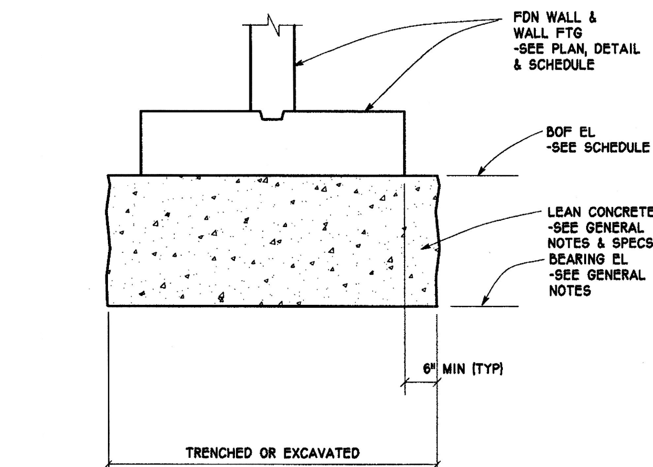
3 TYP 1/2" = 1'-0"
