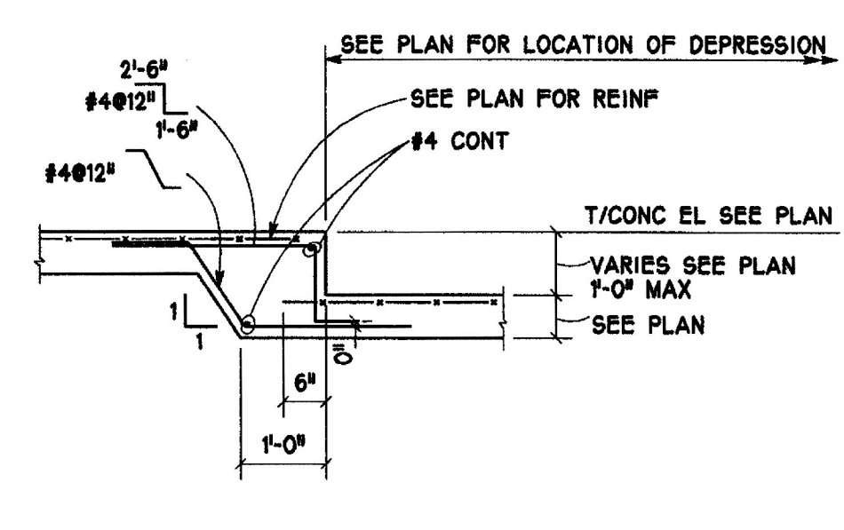
11 TYP NTS
