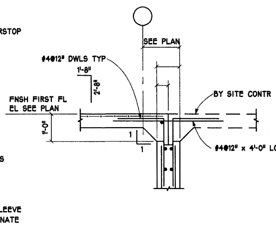
12 TYP NTS
