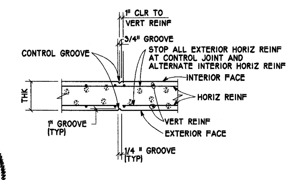
9 TYP NTS
