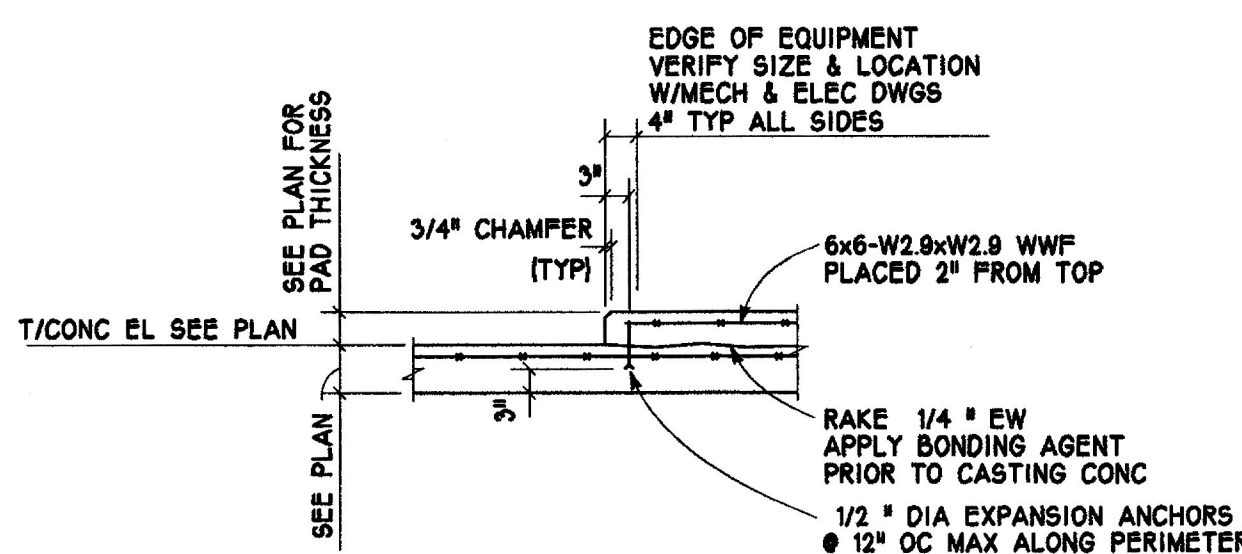
8 TYP NTS
