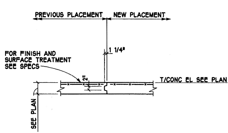
6 TYP NTS
