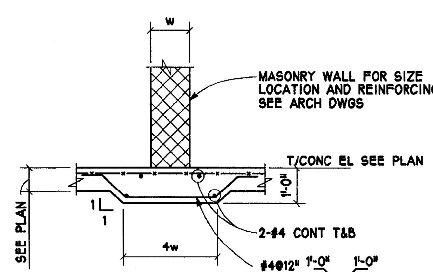
7 TYP NTS
