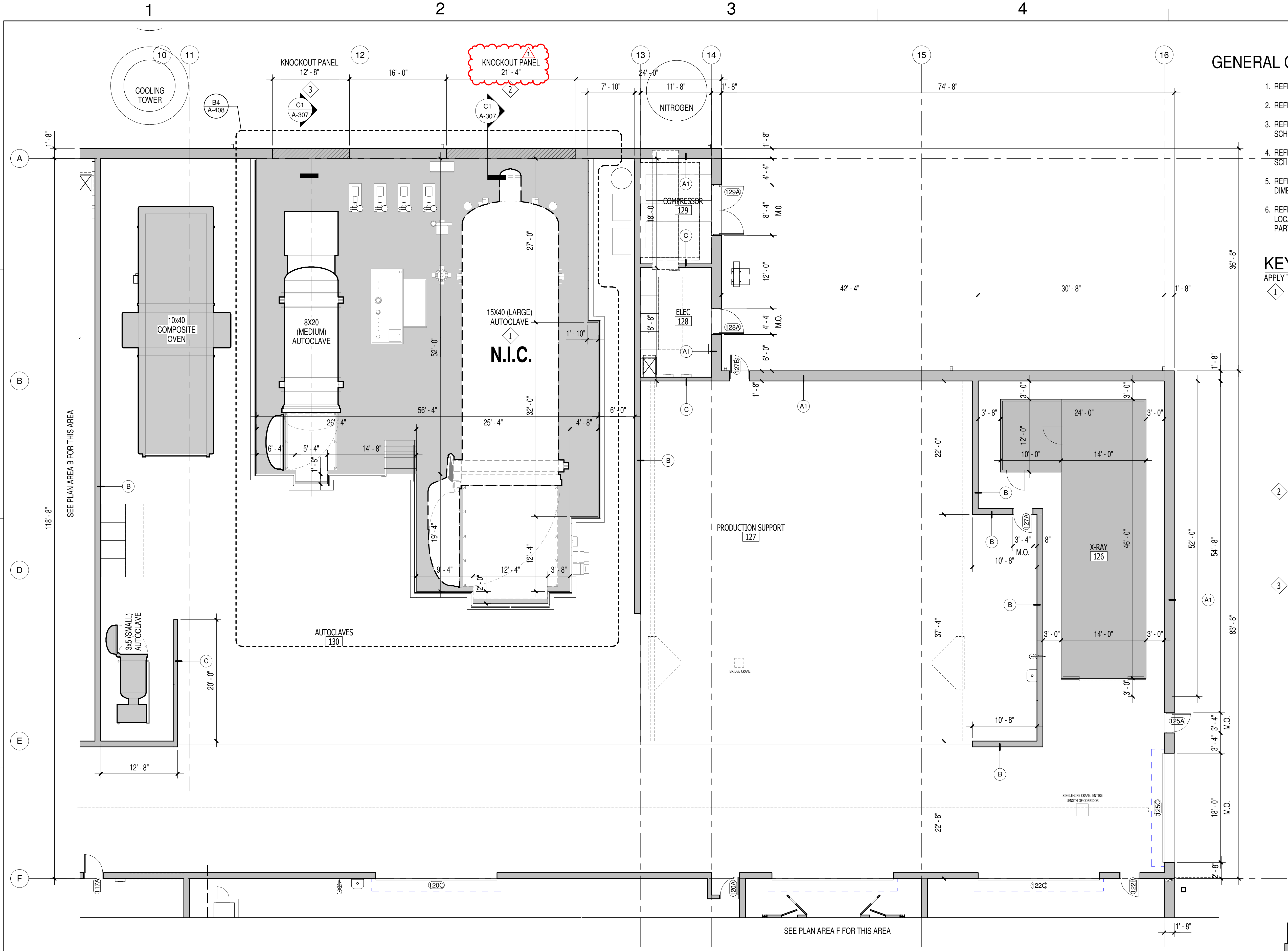
A1 FLOOR PLAN - AREA C SCALE: 1/8" = 1'-0"
