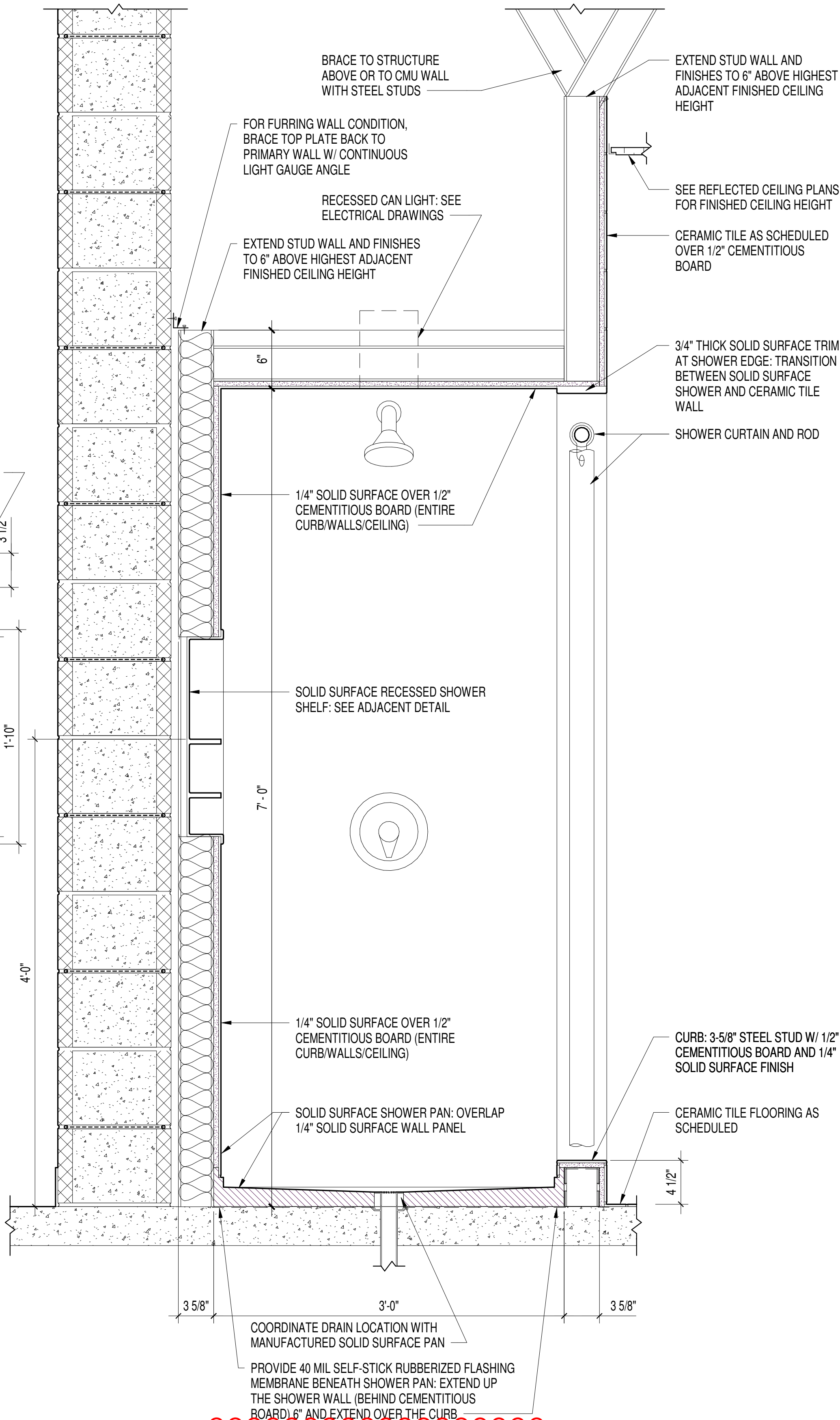
A5 SHOWER SECTION SCALE: 1 1/2" = 1'-0"
