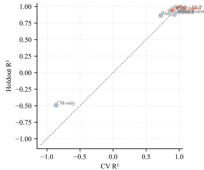
(d) CV vs Holdout Calibration
