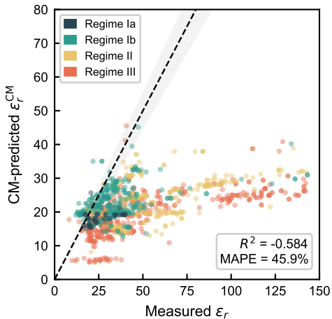
a Clausius–Mossotti fails
