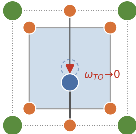
(b) Soft-mode displacement \delta_{\text{LST}} Lyddane-Sachs-Teller enhancement
