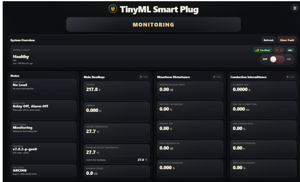
Figure 3.5. Actual PWA live dashboard.
