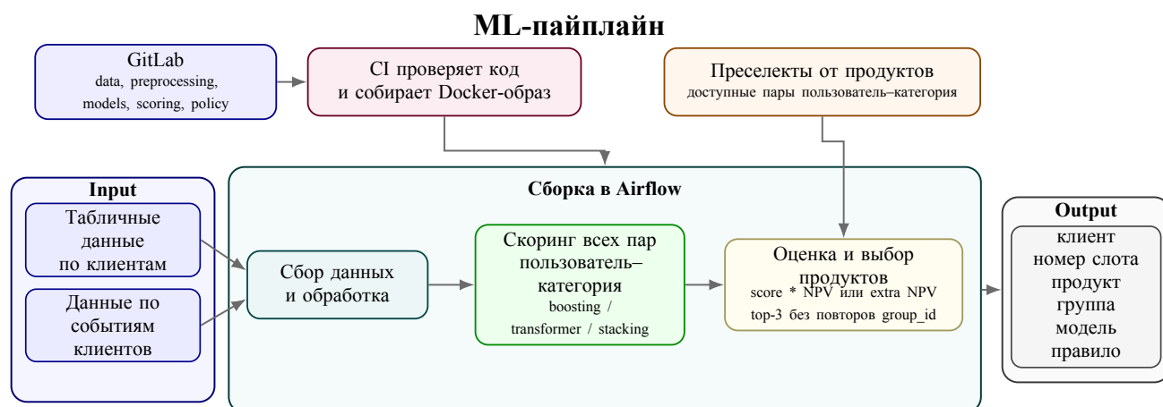
Рис. 1: Инженерный контур расчета: код хранится в GitLab, CI собирает запускаемую версию, Airflow собирает данные, рассчитывает прогнозы и применяет правила выбора категорий.
