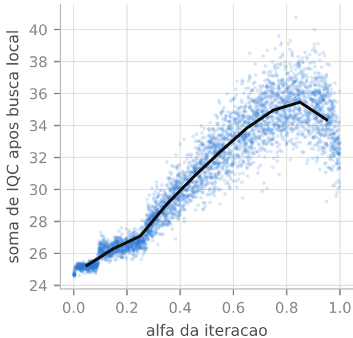
Itajuba / adulto (rho medio +0.91)
