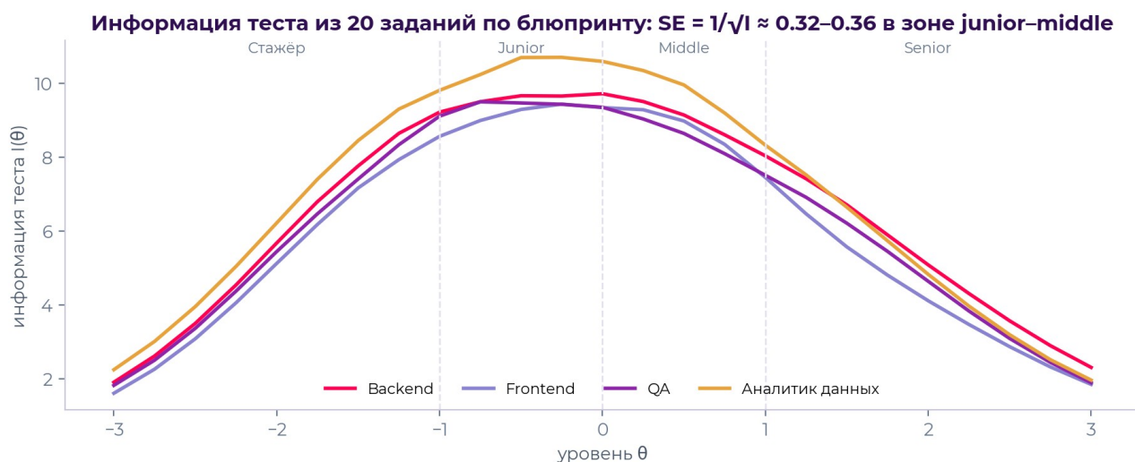
Рисунок 8. Информационная функция теста по специализациям
