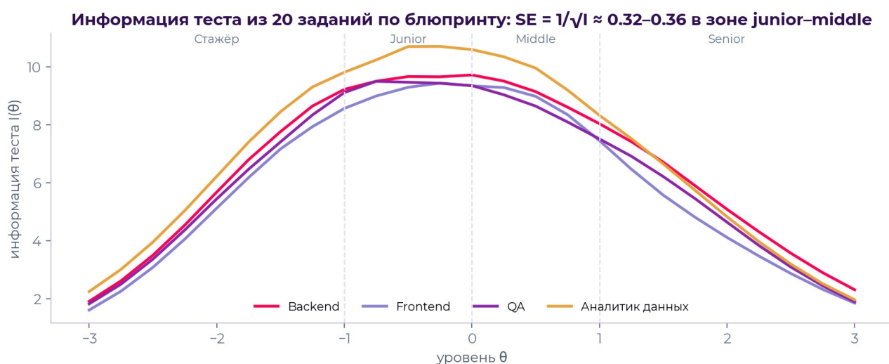
Рисунок 6. Информационная функция теста по специализациям
