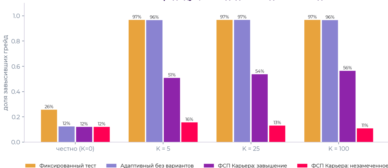
Рисунок 7. Атака «слитой базой»: доля завысивших грейд
