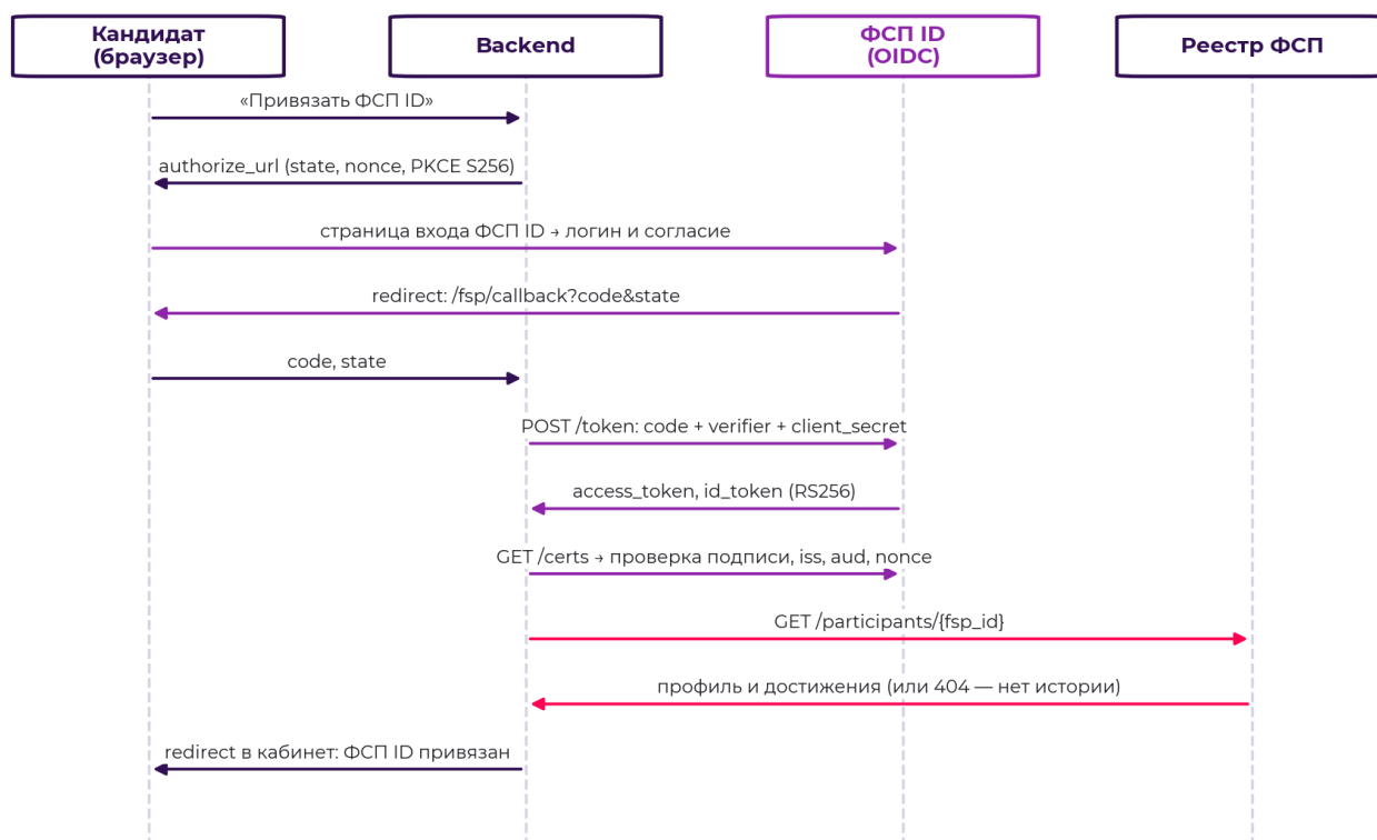
Рисунок 14. Последовательность привязки ФСП ID: OIDC authorization code + PKCE, проверка id_token, загрузка участника из реестра
