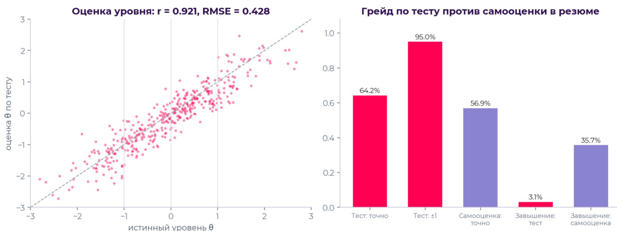
Рисунок 10. Оценка уровня против истинного и сравнение грейда по тесту с самооценкой
