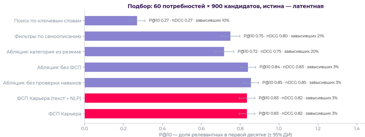
Рисунок 13. Доля релевантных кандидатов в первой десятке по системам
