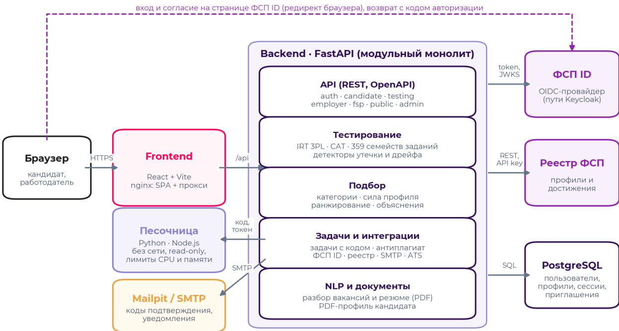
Рисунок 1. Компонентная архитектура: браузер, фронтенд на nginx, модульный монолит на FastAPI, песочница для кода, PostgreSQL, ФСП ID, реестр ФСП, SMTP
