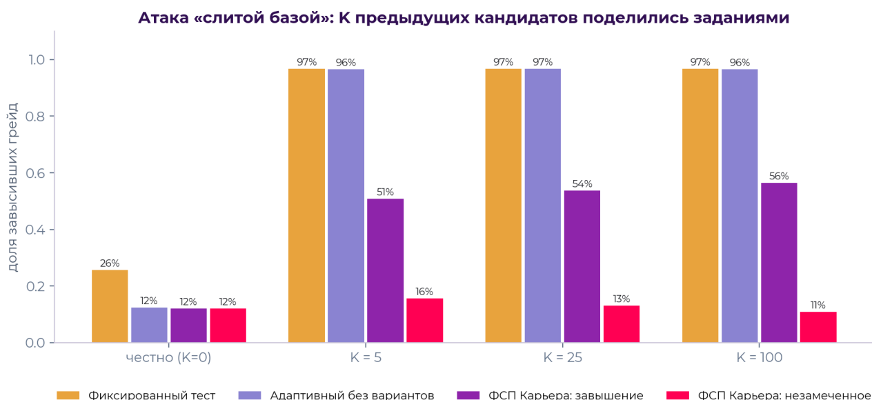
Рисунок 12. Атака «слитой базой»: доля завывсивших грейд
