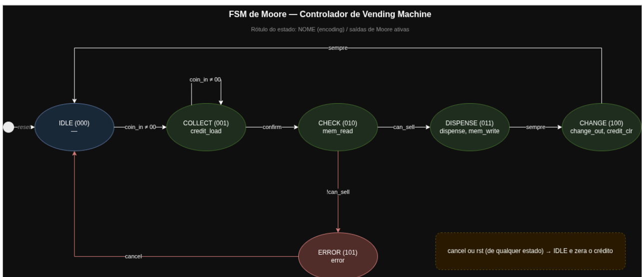
Figura 2 — Diagrama de estados: FSM de Moore, 6 estados (IDLE, COLLECT, CHECK, DISPENSE, CHANGE, ERROR).
