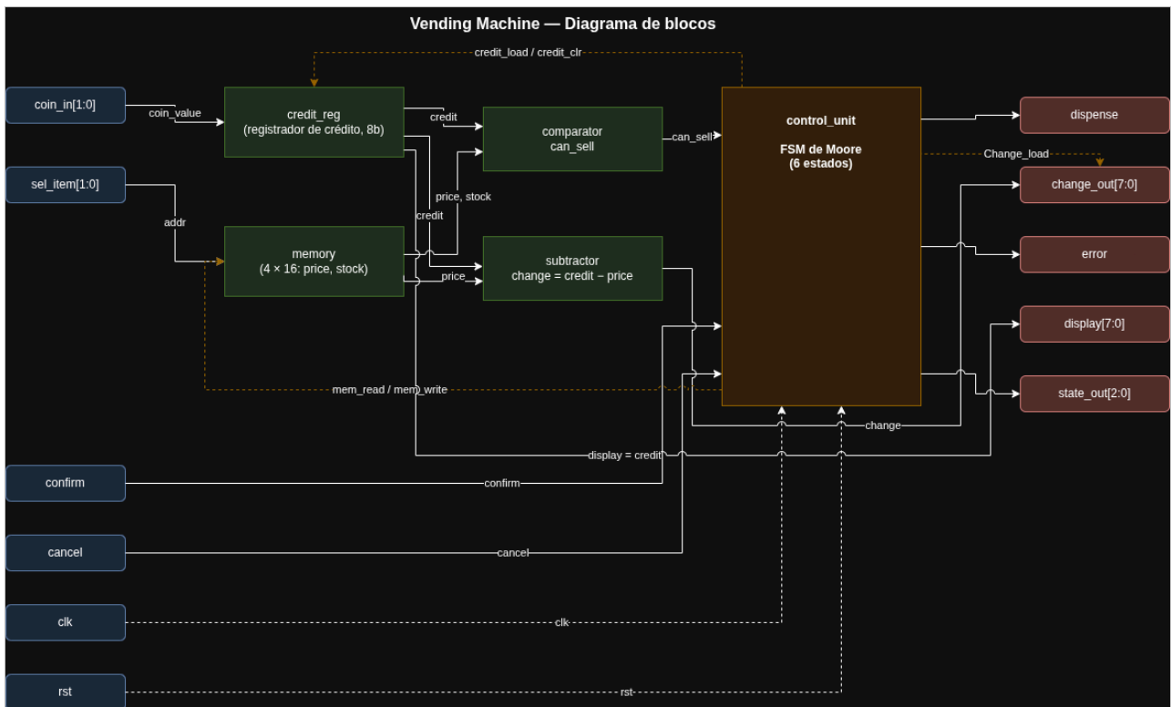
Figura 1 — Diagrama de blocos: entradas → credit_reg, memory, comparator, subtractor, control_unit (FSM) → saídas.
