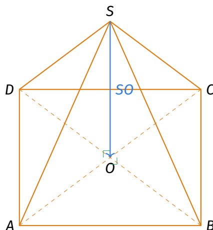
Pyramide régulière SABCD : (SO) hauteur, orthogonale à la base (ABCD)
