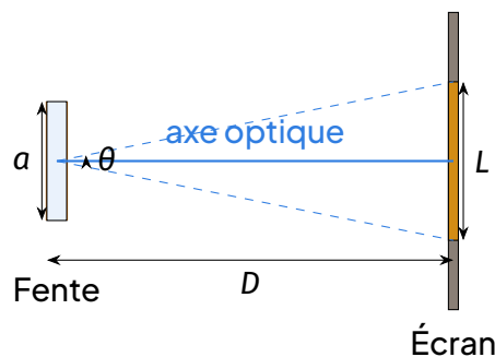
Dispositif de diffraction par une fente : géométrie de la tache centrale.
