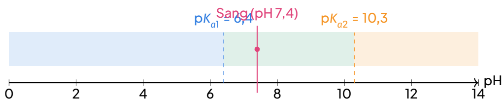
Diagramme de prédominance du système carbonaté (échelle de pH).
