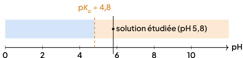
Diagramme de prédominance du couple \text{CH}_3\text{COOH}/\text{CH}_3\text{COO}^- .
