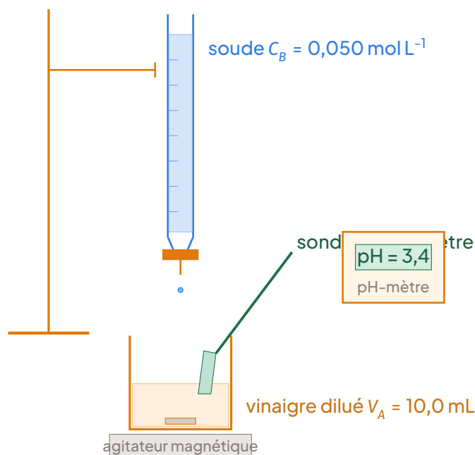
Dispositif de dosage pH-métrique du vinaigre dilué par la soude.
