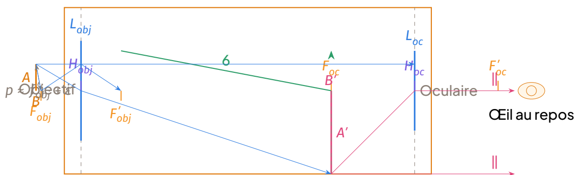
Fonctionnement normal : image finale à l'infini
