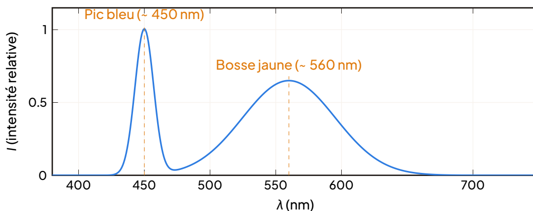
Profil spectral typique d'une DEL blanche : un pic étroit dans le bleu (émetteur InGaN) et une large bosse dans le jaune (luminophore YAG :Ce).
