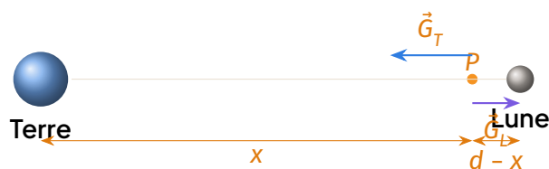
Point d'équilibre gravitationnel Terre–Lune.
