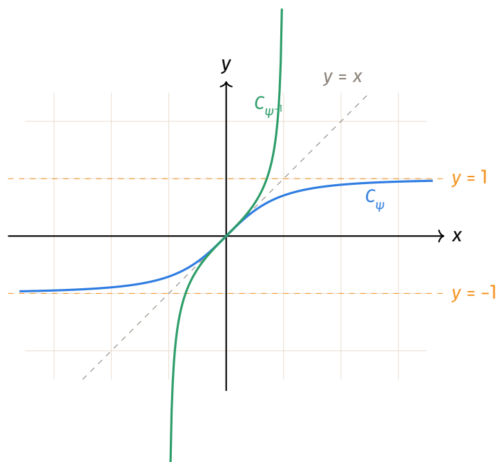
Courbes de \psi et de \psi^{-1} , symétriques par rapport à y = x
