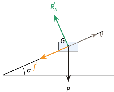
Bilan des forces sur le cartable glissant sur le plan incliné.
