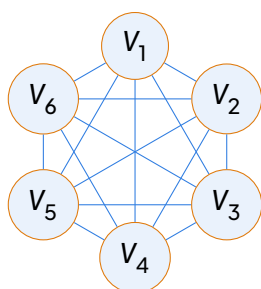
Scénario 1 : K_6 (15 lignes)
