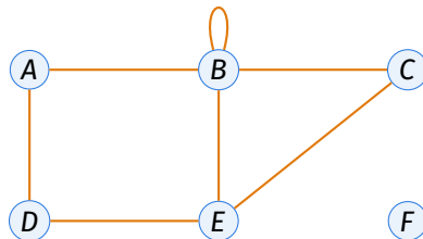
Graphe G : le sommet F est isolé
