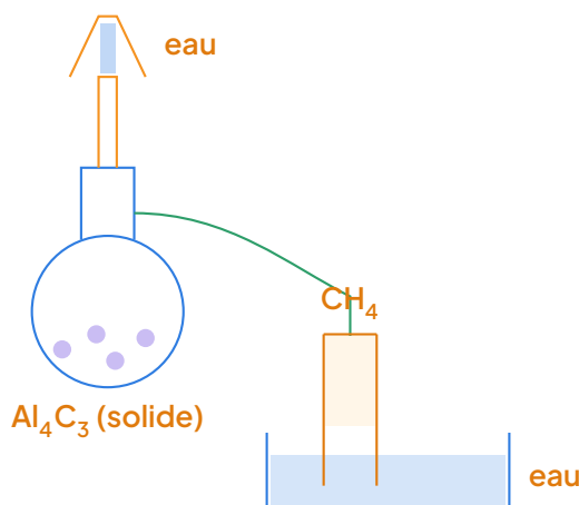
Préparation du méthane par hydrolyse du carbure d'aluminium et recueillement par déplacement d'eau.
