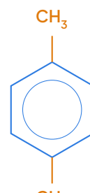
1,4-diméthylbenzène para-xylène
