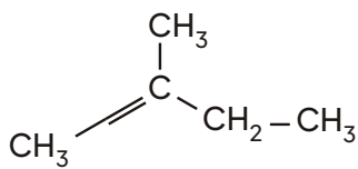
(Z)-pent-2-ène
