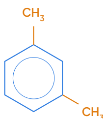
1,3-diméthylbenzène méta-xylène
