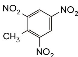
TNT : 2,4,6-trinitrotoluène
