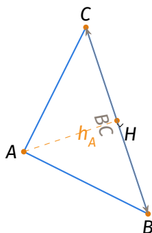
Triangle ABC et hauteur issue de A sur (BC).
