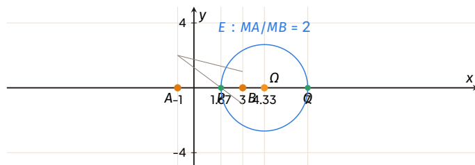
Cercle d'Apollonius pour k = 2 . Centre \Omega milieu de [PQ] , P, Q points de rapport 2 sur (AB) .
