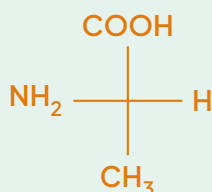
Énantiomère 1
