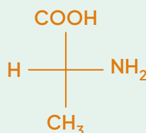
Énantiomère 2
