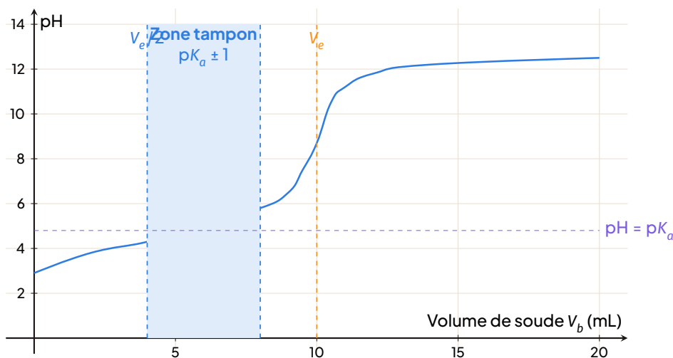
Courbe de dosage d'un acide faible par une base forte : zone tampon (bleu) autour de la demi-équivalence ( V_e/2 ), \text{pH} = \text{pK}_a (violet), saut à l'équivalence V_e (orange).
