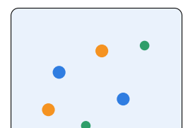
Catalyse homogène une seule phase \text{Fe}^{3+} + \text{I}^- / \text{S}_2\text{O}_8^{2-}
