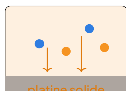
Catalyse hétérogène deux phases \text{Pt (s)} + \text{H}_2/\text{O}_2 \text{ (g)}
