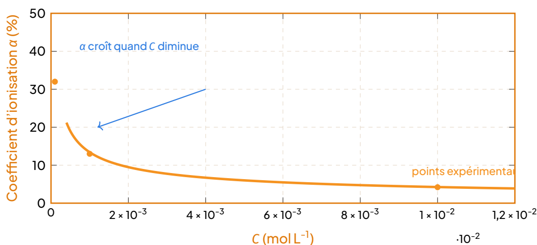
Coefficient d'ionisation \alpha de l'acide éthanöique en fonction de la concentration C : illustration de la loi d'Ostwald.
