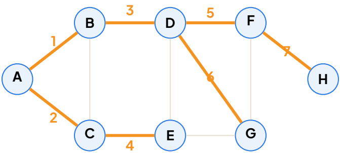
Graphe à 8 sommets. En gras orange : l'arbre BFS depuis A (arêtes de première visite); les numéros indiquent l'ordre de découverte des sommets (A est l'étape 0).
