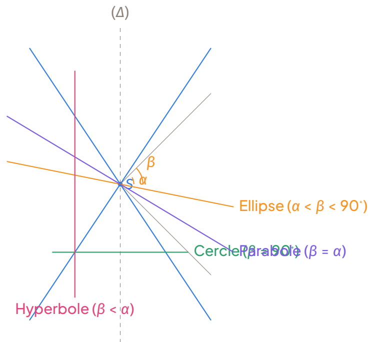
Sections planes d'un cône de révolution : les quatre types de coniques.
