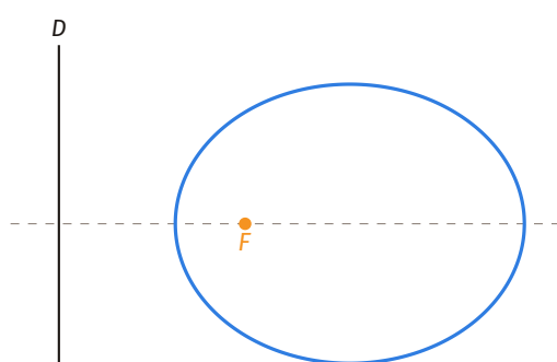
Ellipse : e = 0,6
