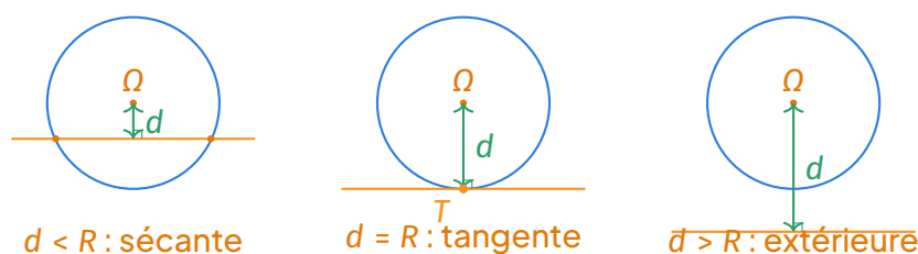
Les trois positions relatives d'une droite (D) et d'un cercle C(\Omega, R) , décidées par la comparaison de d(\Omega, D) et de R .
