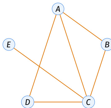
Graphe G des incompatibilités (une arête = une incompatibilité)
