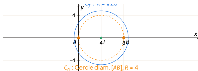
Famille des cercles C_k pour A(0,0), B(8,0) .
