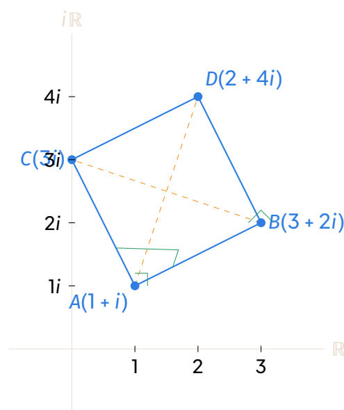
Le carré ABDC construit sur le triangle rectangle isocèle ABC .
