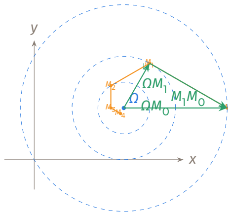
Convergence spiralaire de la suite (M_n) vers le centre \Omega (Exercice 3, Bac).
