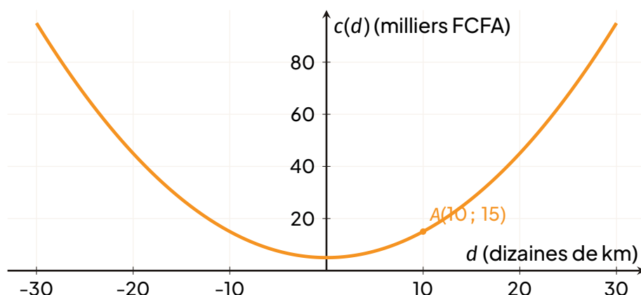
Courbe du coût hebdomadaire d'entretien c(d) = 0,1d^2 + 5 sur [-30; 30] .
