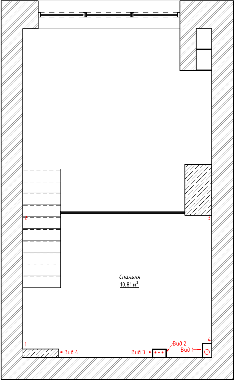
Схема развертки стен. 2 этаж
