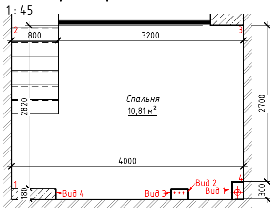
Схема развертки стен. Спальня
