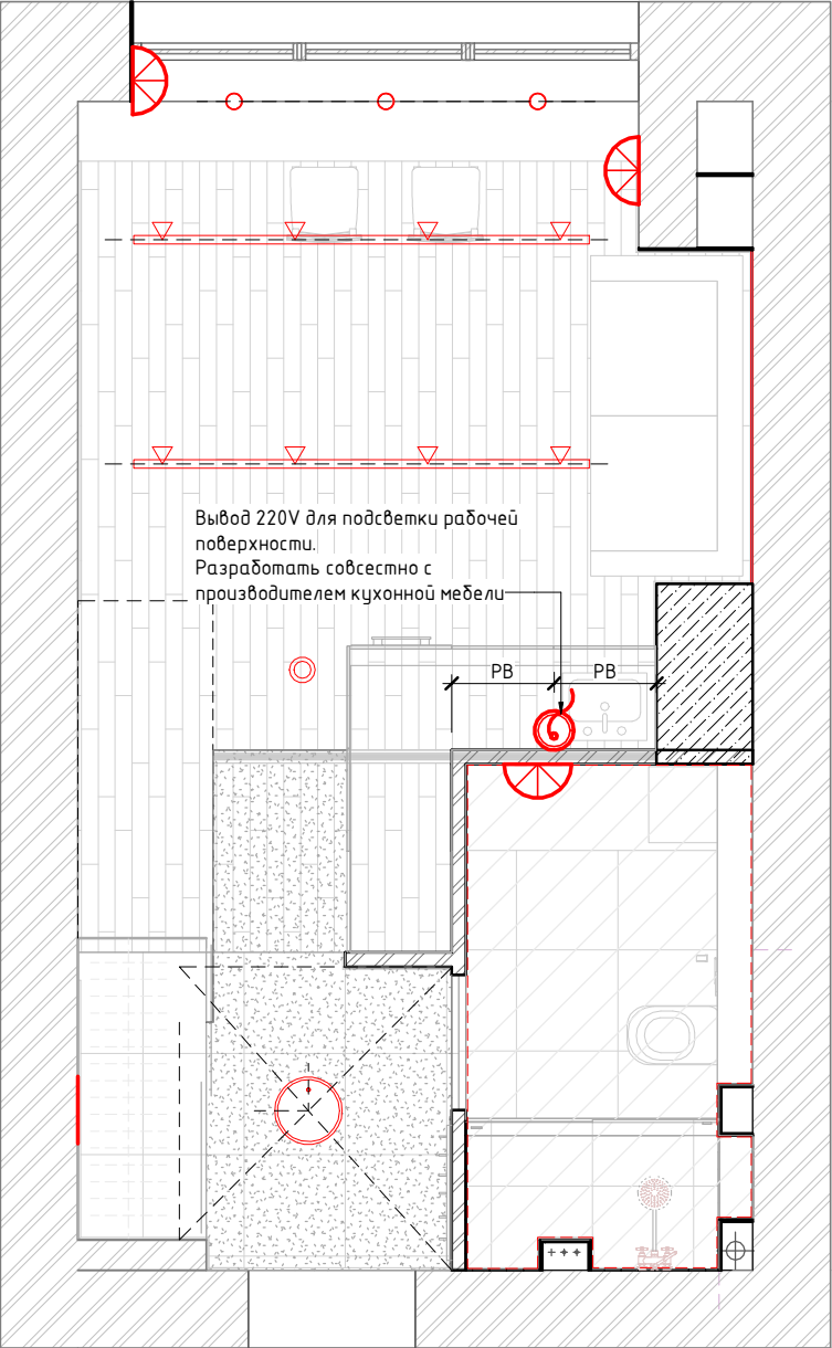
План осветительного оборудования с мебелью. 1 этаж 1 : 35
