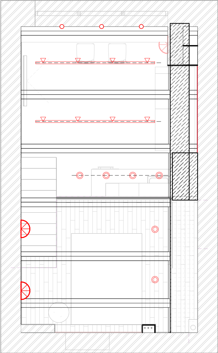
План осветительного оборудования с мебелью. 2 этаж 1 : 35
