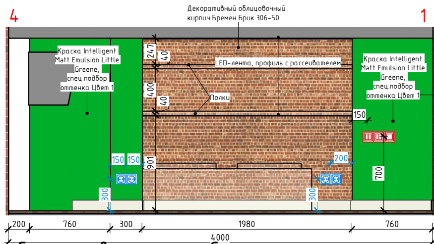
Схема развертки стен. Спальня
