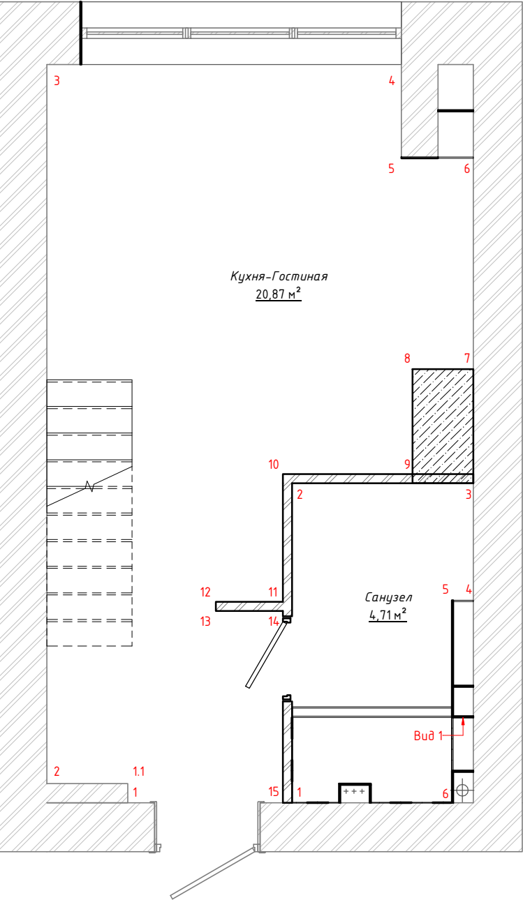
Схема развертки стен. 1 этаж
